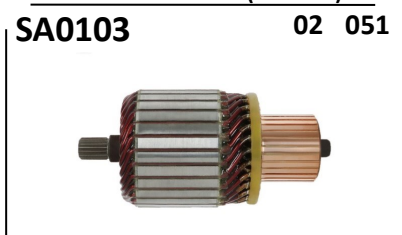
INDUZIDO M/A 12V BOSCH 1004011325 =333775 =062000207
