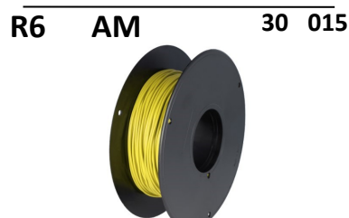
FIO INSTALACAO 1.5mm AMARELO ROLO 100m =06AM
